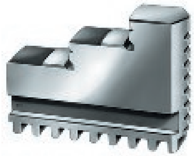
A09 Bohrbacke BB DIN 6350 nach außen abgestufte Backe, gehärtet
