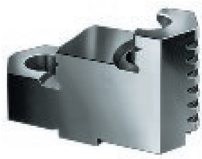
A09 Umkehr-Aufsatzbacken UB DIN 6350 gehärtet Kreuzversatz für Außen- und Innenspannung, Werkstoff 16MnCr5
