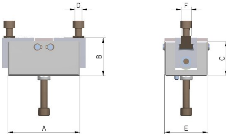
C 15 2-Backen-Greiferfutter GF für Stangenvorschub, für Zylinderschaft DIN 69880 Futter ohne Schaft, ohne Backen
