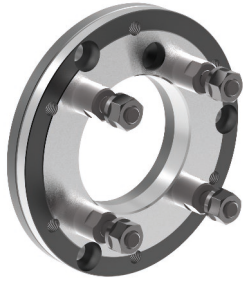
A09 Stahl-Zwischenflansche nach DIN ISO 702-3 (DIN 55027) / Zylindrische Aufnahme futterseitig nach DIN 6350
