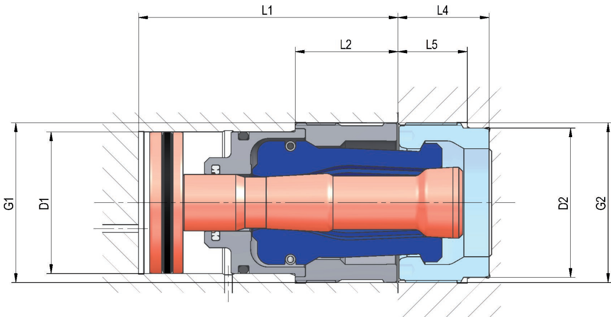
C 15 Einbauspannkopf RESK Wechselschnittstelle zu Maschinenkomponenten
