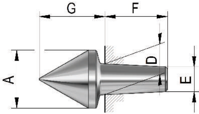
Werkzeuggruppe A06 Auswechselbare Einsätze 60°
