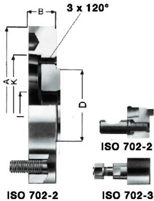
A14 Aufnahme-Flansch Kurzkegel
